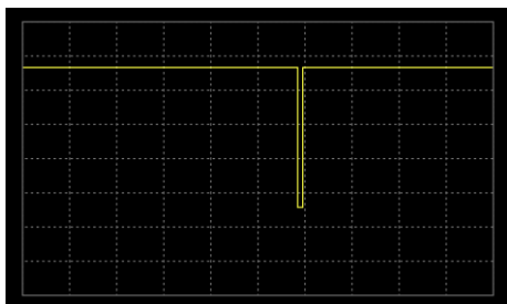
SEQ7 12V のレベル 1 システムのリセットテスト
