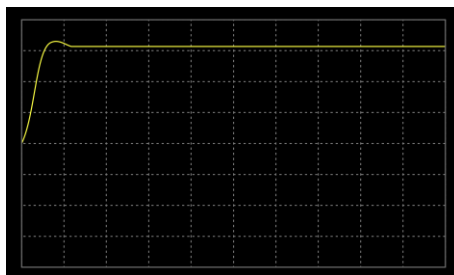
ARB11 2 次ステップ応答 (減衰係数 0.7)
